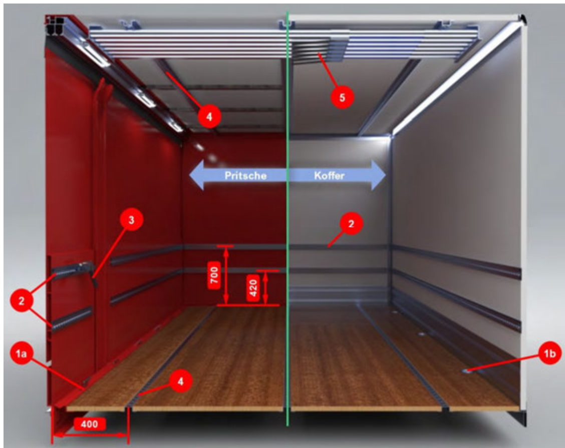
Abbildung 25: Standard-Ladungssicherungskonzept.
