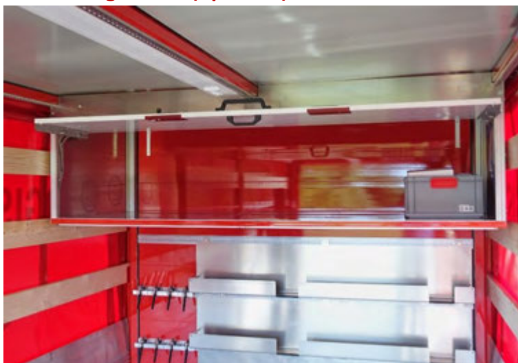
Abbildung 48: Stirnwandeinbauten: Regal und Aufnahme für Bierzeltgarnitur.
