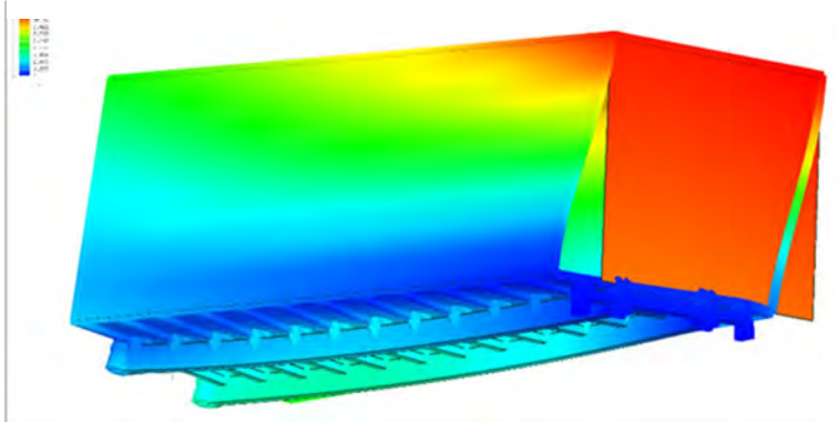
Abbildung 19: FEM-Festigkeitsuntersuchung, hier mit farblich visualisierter Verschiebung und überhöht sichtbar gemachten Verschiebungen in der Struktur, hier Kofferaufbau mit Heckklappe beim virtuellen Verschränkungstest nach DIN.
