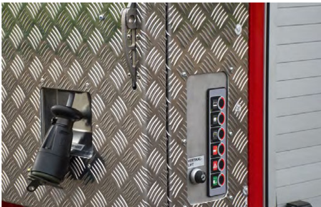
Abbildung 16: Detail – Komfortabler Patentauszug (1.500 mm Auszuglänge) für die Stromversorgung zum Fahrzeug nach DIN. Keine losen Kabel und keine Kabelwicklungen. Der Stecker wird selbsttätig mittels Federauszug eingezogen.
